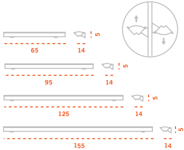
Aplique / Wall lamp / Wandleuchte
