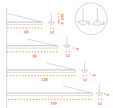
Columna-aplique / Column-wall lamp / Wand-Ausleger-Leuchte
