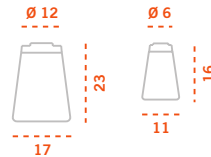
Regleta / track / schiene (WAKI 11 cm)
