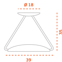
Plafón / ceiling lamp / deckenleuchte
