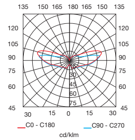
PL 13W
