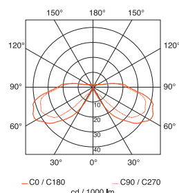
PL 23W
