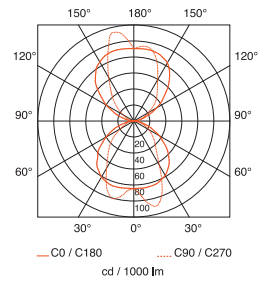
PL 15W
