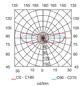
PL 18W
