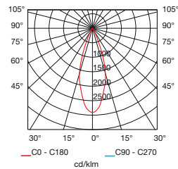
CDM-R111 70W 40D
